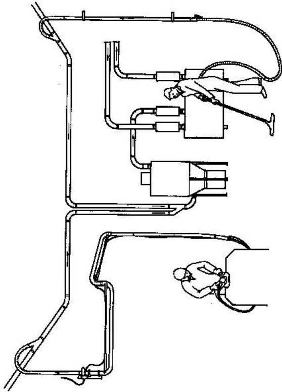
Oplossingenkaart afzuiging handmachines: figuur 5
