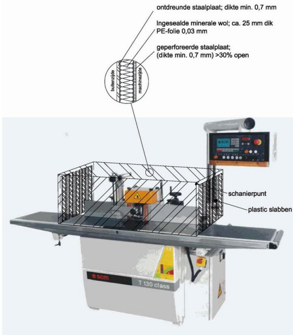
Oplossingenkaart tafelfrees: figuur 1
